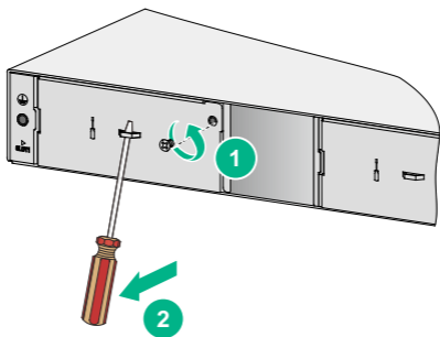
图2 拆卸假面板
