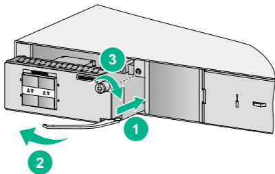
图3 安装 LSWM2SP4P-Z 示意图
