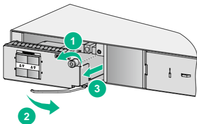
图4 拆卸 LSWM2SP4P-Z 示意图
