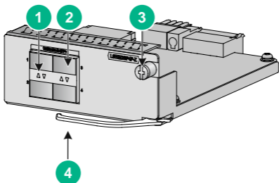
图1 LSWM2SP4P-Z 外观图
